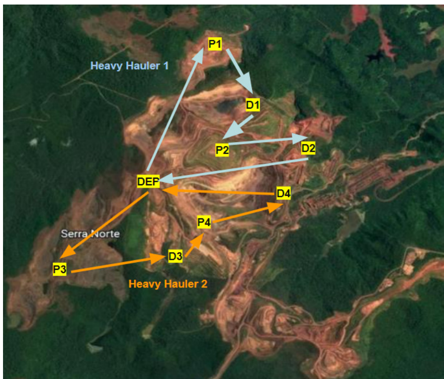
Figura 3.1: Exemplo de solução para dois caminhões prancha
